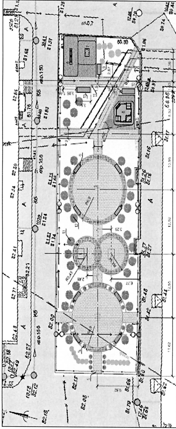
План благоустройства, М. 1:200 Вид с юга 1
