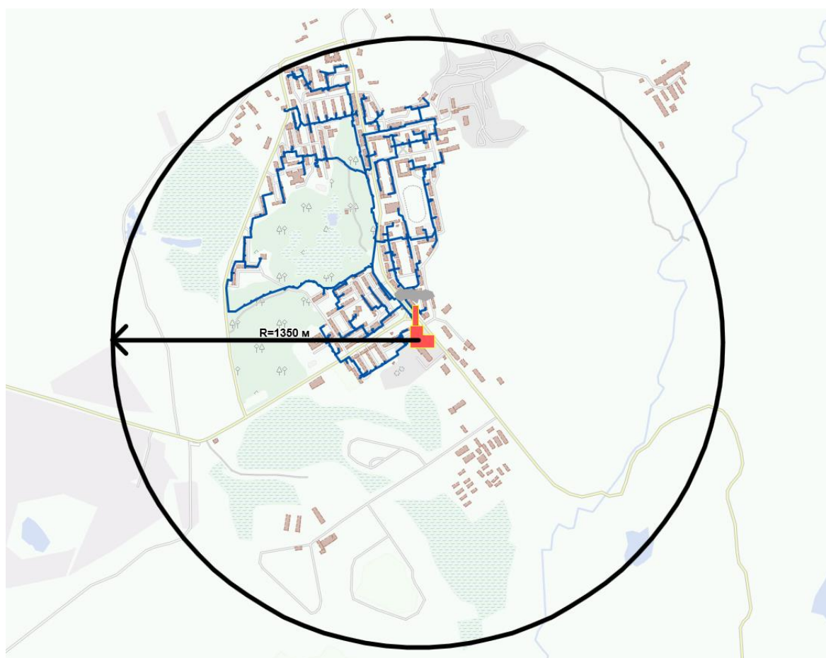
Рисунок 5 - Радиус эффективного теплоснабжения
