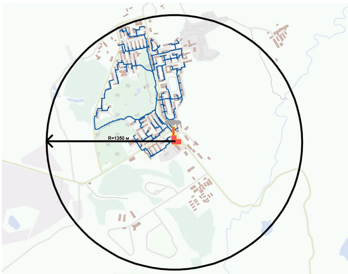
Рисунок 1 - Радиус эффективного теплоснабжения
